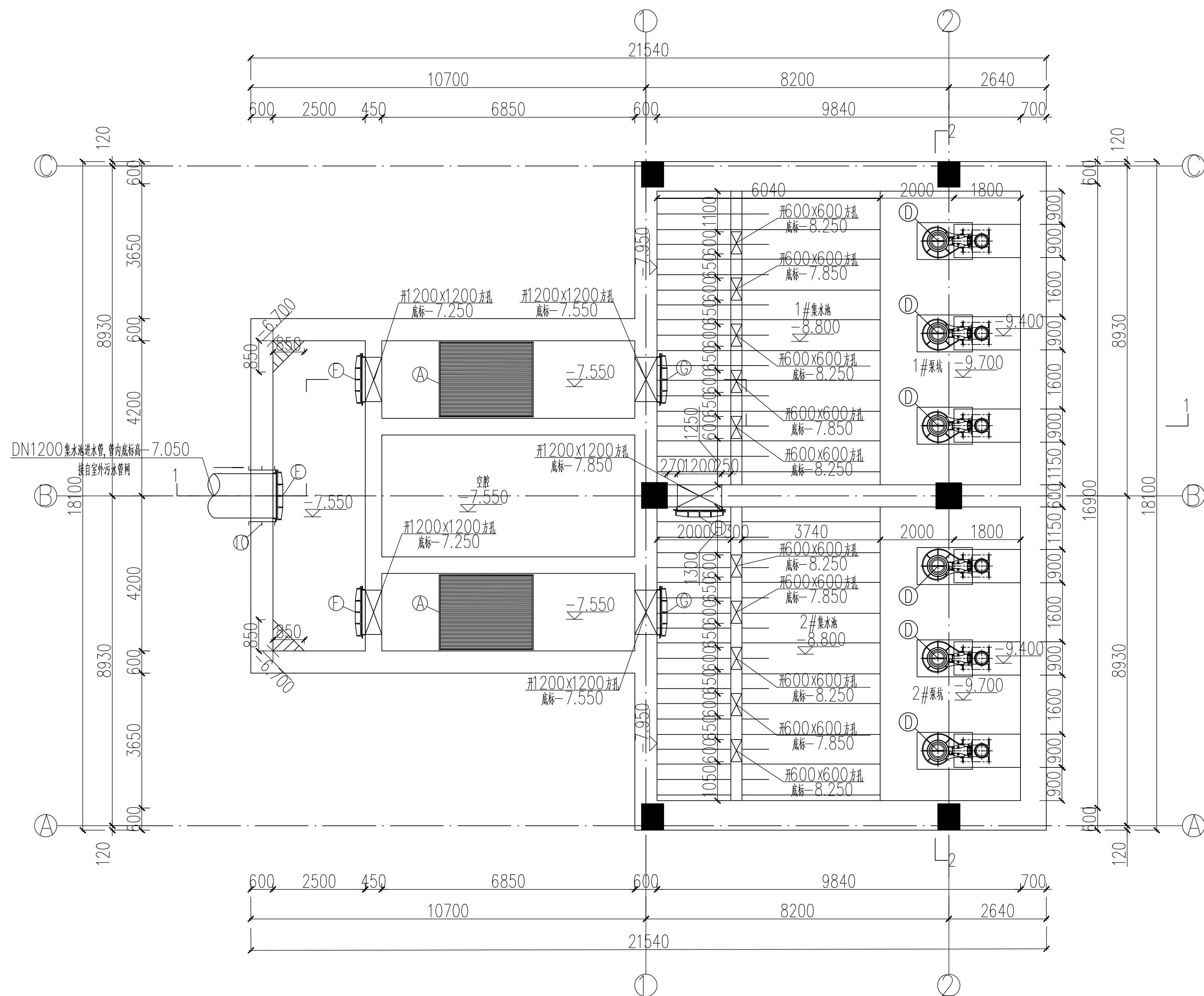
集水池及提升泵站—6.000m 标高管线布置平面图 1:100
