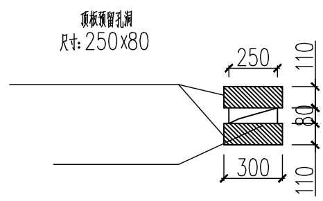
编号G 明杆式不锈钢方闸门b向大样图 1:25
