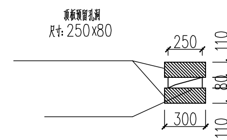
编号H 明杆式不锈钢方闸门b向大样图 1:25
