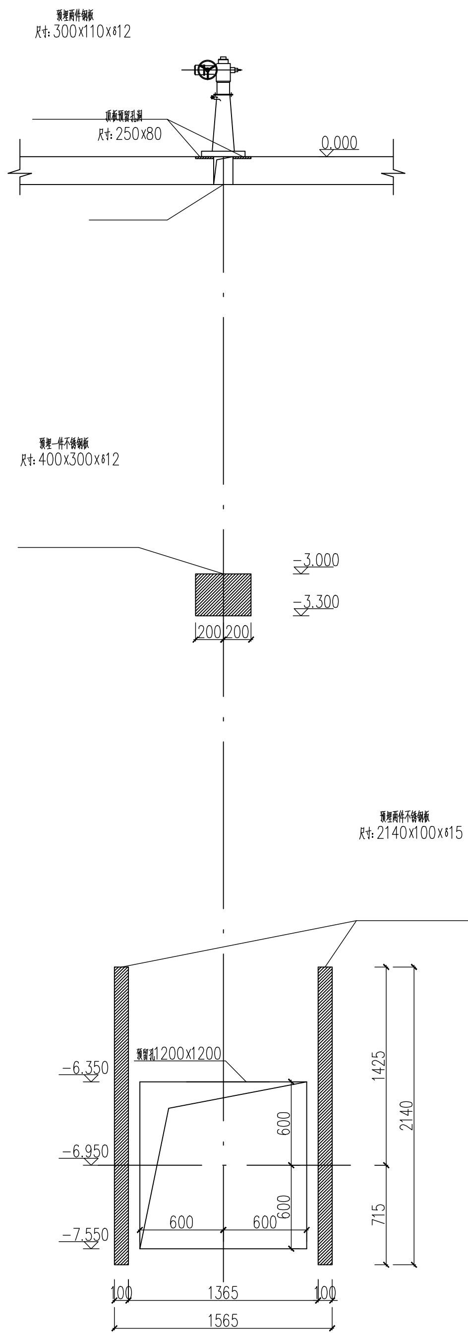
编号G 明杆式不锈钢方闸门a向大样图 1:25
