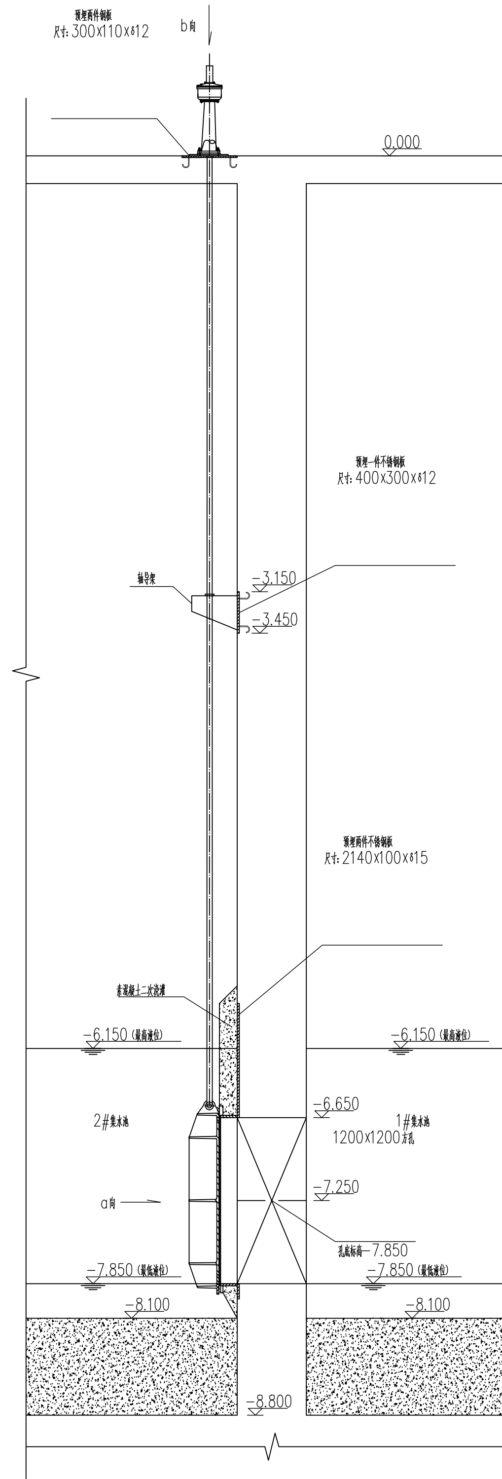
编号H 明杆式不锈钢方闸门安装详图 1:25
